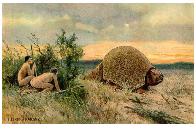
čtvrtohory
