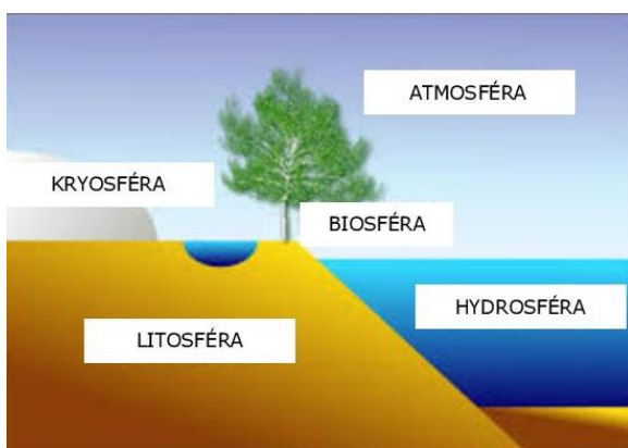
sféry Země
