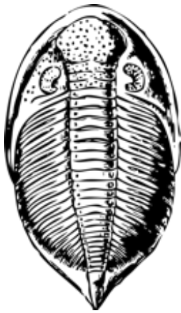
trilobit
